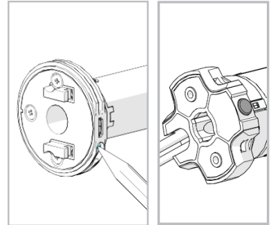
Bouton P1 sur la tête du moteur.
